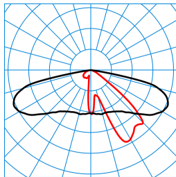
Publisca P1-AB2L-LR/1000-730 2G1S TX047503 ■ C0 - C180 ■ C90 - C270 DIN 5040: A30 UTE: 1,00 G CEN Flux Code: 34 70 96 100 100
