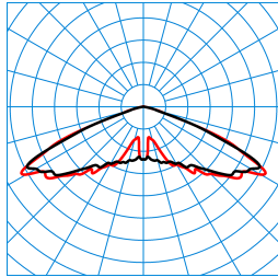
Publisca P1W-RB6L-LR/1800-730 2G1S ET (CLO end value) TX301350
