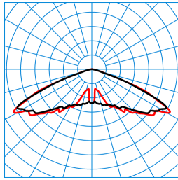
Publisca P1W-RB6L-LR/1800-730 2G1S ET (CLO initial value) TX300773
