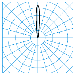
Altigo G2 10 RE1L/350-830 1G1P + G2 VE IP66 24V DC 120W TX113640
