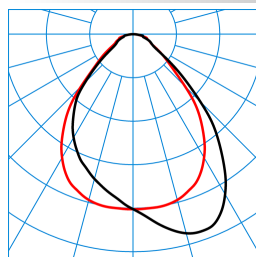
ArimoFit G2 M57 P-WW 42-840 ET TX376498
