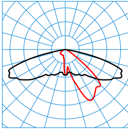
Publisca P1W-AB2L-LRA/3800-740 6G1S TX053504
