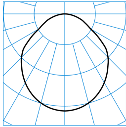
Inplana C07 OTA22 1000-840 01 + C07 ZPF - T WR TX045468
