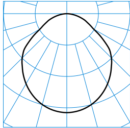
Inplana C07 OTA22 1000-840 01 + C07 ZPF - T TX045467
