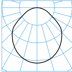
Inplana C07 OTA22 1000-840 ETDD 01 TX372434
