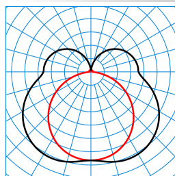
7131 O 1200 LED3000-830 TX373628
