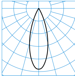
E-Line 7651 Lentyp L-FL 40-827 M32 ET 03 (225) TX463174
