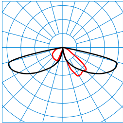
CS 19 100-AB2L-LR/1650-740 2G1S ET (CLO initial value) TX299983
