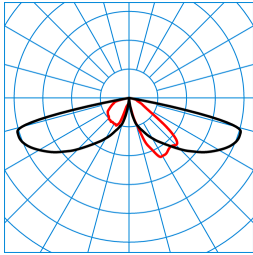
CS 19 100-AB2L-LR/1650-740 2G1S ET (CLO end value) TX299982
