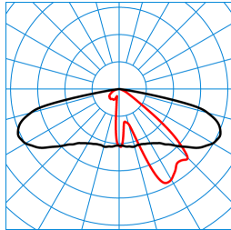
Publisca P1-AB2L/1200-740 2G1S ETDD (CLO end value) TX300889
