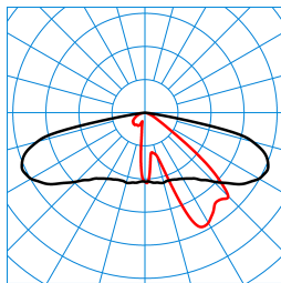
Publisca P1-AB2L/1200-740 2G1S ETDD (CLO initial value) TX300447
