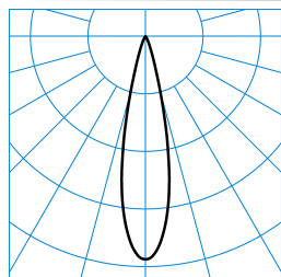
E-Line 7651 LentyP L-SP 20-EC M39 ET 01 (150) TX463525
