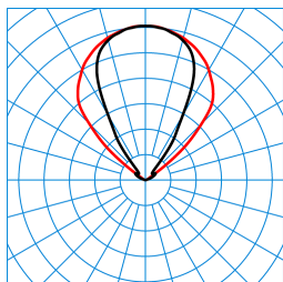
Bicult Act T COM TGCS 5500 I KL 03 EU (ActIWW) TX095983 DIN 5040: E04 UTE: 0,00 J + 1,00 T CEN Flux Code: 0 0 0 0 100 82 96 100 100 ■ C0 - C180 ■ C90 - C270
