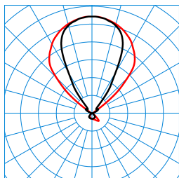
Bicult Act T COM TGCS 5500 I KL 03 EU (ActCCW) TX095975 DIN 5040: D54 UTE: 0,10 D + 0,90 T CEN Flux Code: 59 89 98 10 100 82 96 100 90 ■ C0 - C180 ■ C90 - C270
