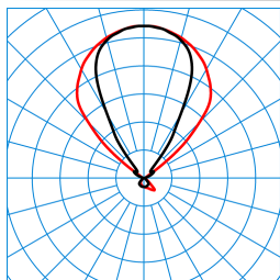
Bicult Act T COM TGCS 5500 I KL 03 EU (ActCWW) TX095977 DIN 5040: D54 UTE: 0,10 D + 0,90 T CEN Flux Code: 59 89 98 10 100 82 96 100 90 ■ C0 - C180 ■ C90 - C270
