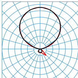
LuceoS S-T PAW-IL 300-830 01(LEO1) TX372006
