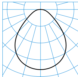
Inplana C07 CDP19 1000-830 01 + C07 ZPF - T TX045461
