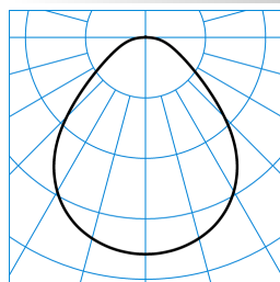
Inplana C07 CDP19 1000-830 ETDD 01 TX373825
