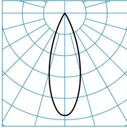
E-Line 7651 Lentyp L-FL 40-EW M48 ET 05 (225) TX463154
