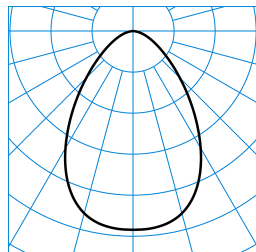
InperiaL G2 C07 HR19 2700-840 03 + DA-M 03 ■ C0 - C180 TX373370
