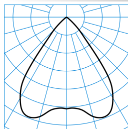
InperiaL G2 C07 HR19 2700-840 03 ■ C0 - C180 TX373373
