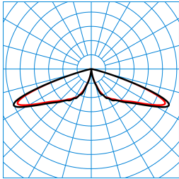
CS 19 100-RB6L-SLR1/5100-740 4G1S ET (CLO initial value) TX300142
