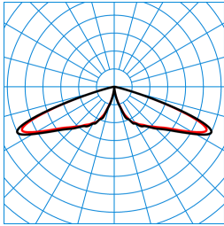
CS 19 100-RB6L-SLR1/5100-740 4G1S ET (CLO end value) TX300141
