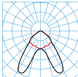
7651 LightP DA-B-DA 65-830ET L75 03 (225) TX557613
