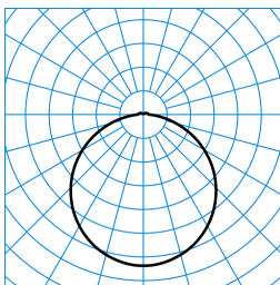
Olisq RWD2 DW 20-830 ETBLE +DMM IP54 PC + Olisq RWD2 C 01 TX425765
