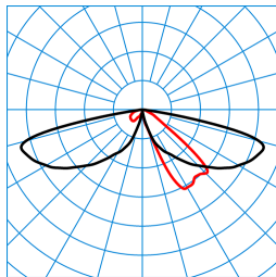
LTX P-AB2L-LRA/15/18/26-730 4G1 (1800 lm) TX062699
