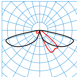
LTX P-AB2L-LRA/15/18/26-730 4G1 (2600 lm) TX062700
