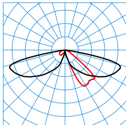
LTX P-AB2L-LRA/15/18/26-730 4G1 (1500 lm) TX059698
