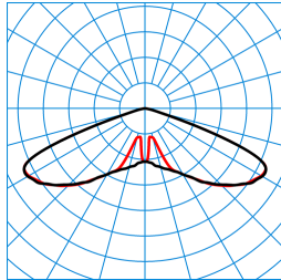
Publisca P1-RB6L/1000-740 2G1S ETDD (CLO end value) TX301166
