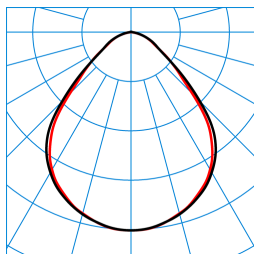
Opendo D2-L PW19 20-47/5/ML-840 ET 03 (3100lm) TX376539
