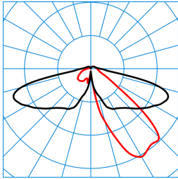
8841LS-UE 260-AB2L/1000-740 2G2 ET (CLOANFANGSWERT) TX369490
