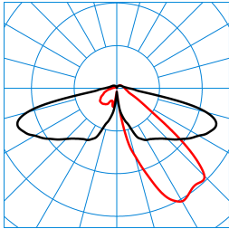
8841LS-UE 260-AB2L/1000-740 2G2 ET (CLOENDWERT) TX369369
