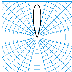
Altigo G2 60 WO RM3L/2000-830 1G1P + G2 VE IP66 24V DC 30W TX113722 ■ C0 - C180 DIN 5040: E04 UTE: 0,00 J + 1,00 T CEN Flux Code: 0 0 0 0 100 97 99 100 100
