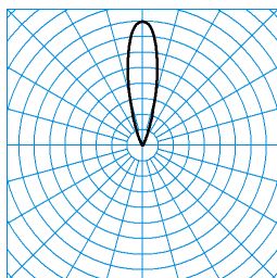
Altigo G2 60 WO RM3L/2000-830 1G1P + G2 VE IP66 24V DC 80W TX113723 ■ C0 - C180 DIN 5040: E04 UTE: 0,00 J + 1,00 T CEN Flux Code: 0 0 0 0 100 97 99 100 100
