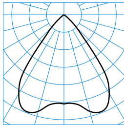
InperiaL G2 C07 HR19 1800-840 01 ■ C0 - C180 TX053013
