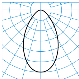
InperlaLP C05 BR19 1800-830 01 + DA-M 01 TX041506 ■ C0 - C180
