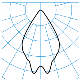
InperlaLP C05 BR19 1800-830 01 + RD-PC TX041508 ■ C0 - C180
