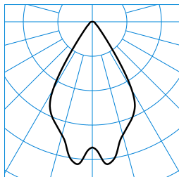
InperlaLP C05 BR19 1800-830 01 + ZN-PC TX041510 ■ C0 - C180
