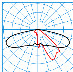
Publisca P2-AB2L/2000-730 3G1S TX047708
