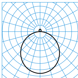
Solegra WD2 OTA 6000-840 + WD2 ZP 03 TX373196
