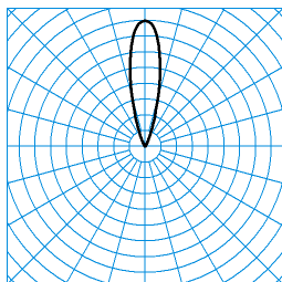
Altigo G2 60 RM3L/2000-830 1G1P + G2 VE IP66 24V DC 120W TX113939
