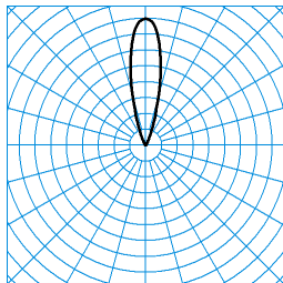
Altigo G2 60 RM3L/2000-830 1G1P + G2 VE IP66 24V DC 240W TX113942 ■ C0 - C180 DIN 5040: E04 UTE: 0,00 J + 1,00 T CEN Flux Code: 0 0 0 0 100 97 99 100 100
