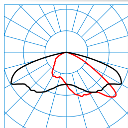
LIQ 70N-AB7L-SLR2/14500-727 12G1 ET (CLO end value) TX278072
