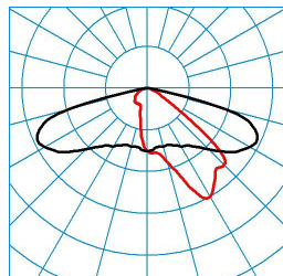
Jovie 50-AB2L-6-68-730-CLO-E
