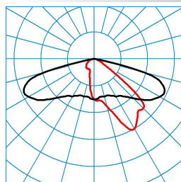
Jovie 50-AB2L-6-68-730-CLO-B
