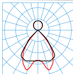
SFlow H3-L MRX LED6400-840 LLWS 01 TX053184
