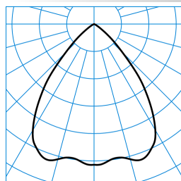
InperiaLP C05 BR22 1000-830 03 TX040944 ■ C0 - C180
