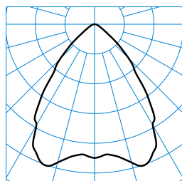
InperiaLP C05 BR22 1000-830 03 + RG-PC TX041535 ■ C0 - C180
