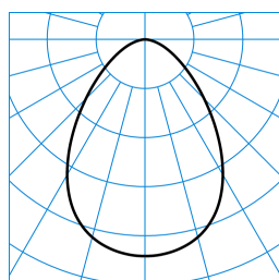
InperiaLP C05 BR22 1000-830 03 + DA-M 01 TX041532 ■ C0 - C180
