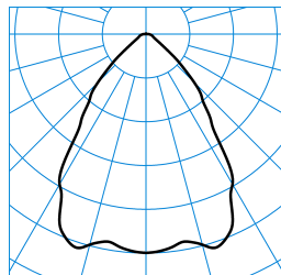
InperiaLP C05 BR22 1000-830 03 + ZN-PC TX041536 ■ C0 - C180
