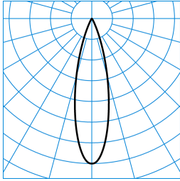
E-Line 7651 LentyP L-MF 40-835 M34 ETDD 05 (225) TX463446
