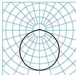
Olisq QWD2 DW 35-830 ET EB3 IK + Olisq QWD2 ZDR 1/2 05 TX461560
