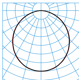
Olisq QWD2 DW 35-830 ET EB3 IK + Olisq QWD2 ZDR 1/1 01 TX460688
