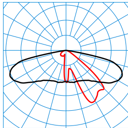
Publisca P1-AB2L-LRA/1000-730 2G1S ET (CLO end value) TX300373 ■ C0 - C180 ■ C90 - C270 DIN 5040: A30 UTE: 1,00 G CEN Flux Code: 34 70 96 100 100
