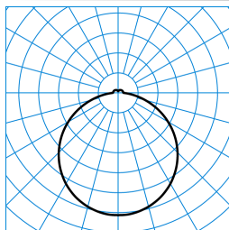
Olisq RWD4 DW 40-840 ET HFS IP54 TX375664
