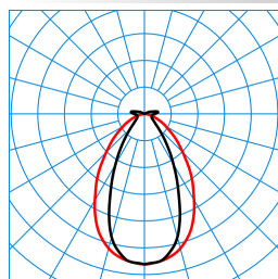
AragF 15 PN 80-840 ETDD CR TX122256
