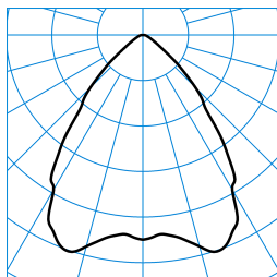
InperiaLP C05 BR22 1800-840 03 + RG-PC TX041554 ■ C0 - C180
