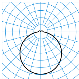
Olisq RWD3 DW 50-830 ETBLE +DMM PC + Olisq RWD3 ZDR 1/2 01 TX426727
