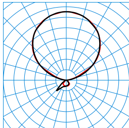
LuceoS S-U PAW-IL 300-830 01(LEO2) TX245491
