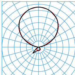
LuceoS S-U PAW-IL 300-830 01(LEO1) TX371976
