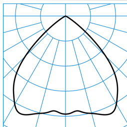
InperiaL G2 C07 HR22 2700-840 03 TX372001 ■ C0 - C180
