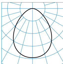
InperiaL G2 C07 HR22 2700-840 03 + DA-M 03 TX372010 ■ C0 - C180
