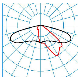
Jovie 50-AB2L-6-51-740-CLO-E
