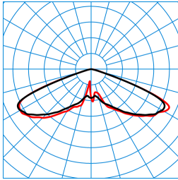
Publisca P1-RB6L-LRA/2000-740 3G1S TX047666 ■ C0 - C180 ■ C90 - C270 DIN 5040: A20 UTE: 1,00 J CEN Flux Code: 20 57 98 100 100
