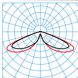
9821 RB6L-LRA/2600-740 3G1S ET TX049022
