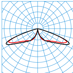
CS 19 100-RB6L-LR/2900-740 2G1S ET (CLO initial value) TX300086
