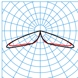
CS 19 100-RB6L-LR/2900-740 2G1S ET (CLO end value) TX300085
