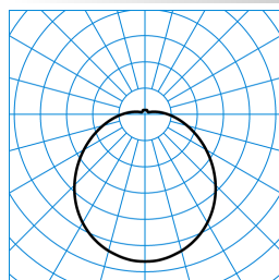
Mondia G3 K WD3 DW 32-840 ET +HFS PC TX390299
