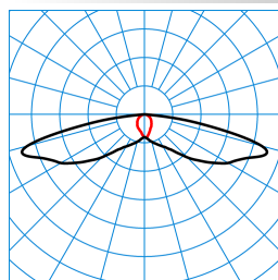
LIQ 50N-SB3L-LR/1000-722 2G1 ET (CLO end value) TX281121
