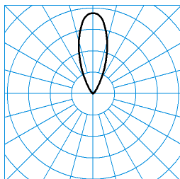
Altigo G2 10 RB17L/300-830 1G1P + G2 VE IP66 24V DC 30W TX113632 ■ C0 - C180
