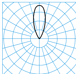
Altigo G2 10 RB17L/300-830 1G1P + G2 VE IP66 24V DC 120W TX113630
