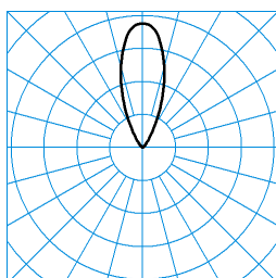
Altigo G2 10 RB17L/300-830 1G1P + G2 VE IP66 24V DC 80W TX113633 ■ C0 - C180
