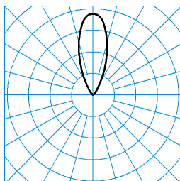
Altigo G2 10 RB17L/300-830 1G1P + G2 VE IP66 24V DC 240W TX113631 ■ C0 - C180
