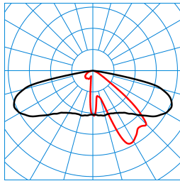
Publisca P1-AB2L-LRA/1200-730 2G1S ET (CLO end value) TX300955 ■ C0 - C180 ■ C90 - C270 DIN 5040: A30 UTE: 1,00 G CEN Flux Code: 34 70 96 100 100
